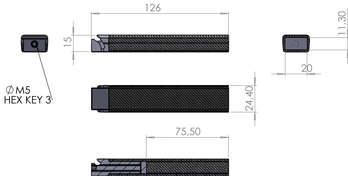
SEZIONE A-A SCALA 1 : 2
